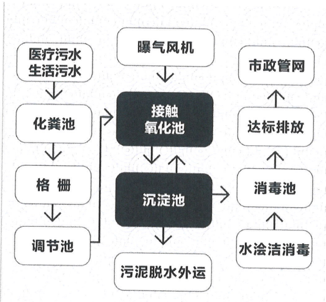
图 1 废水处理流程图
