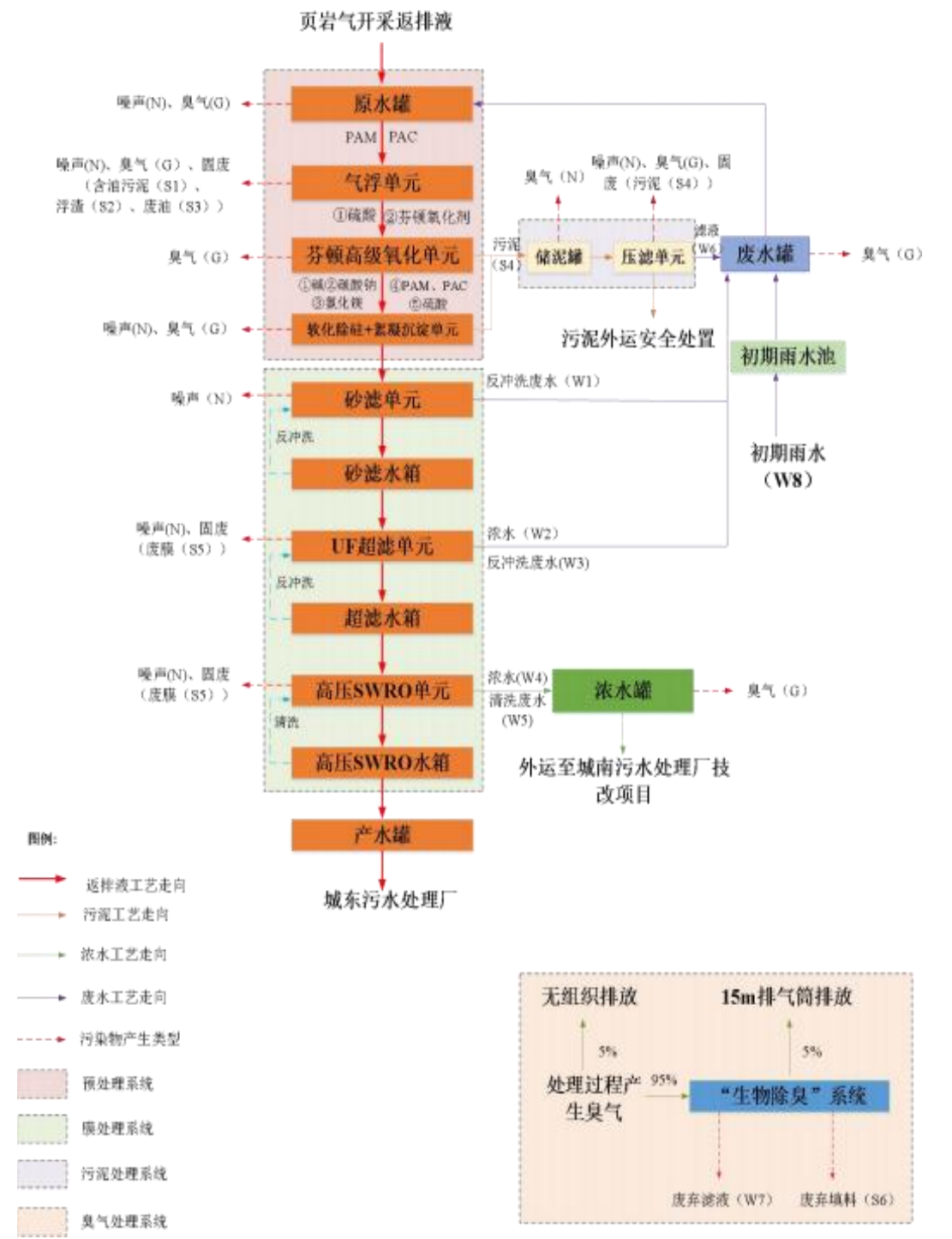
图 3-1 生产工艺及产污流程图
